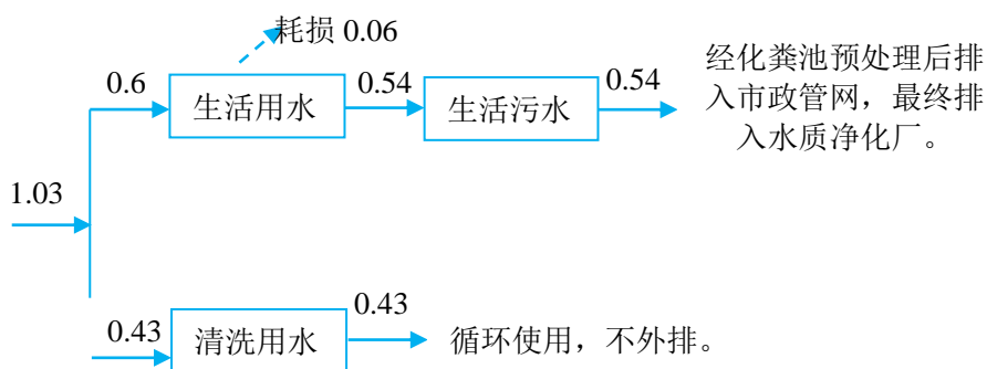
图 2-1 项目用水平衡图 (单位: \text{m}^3/\text{d} )
