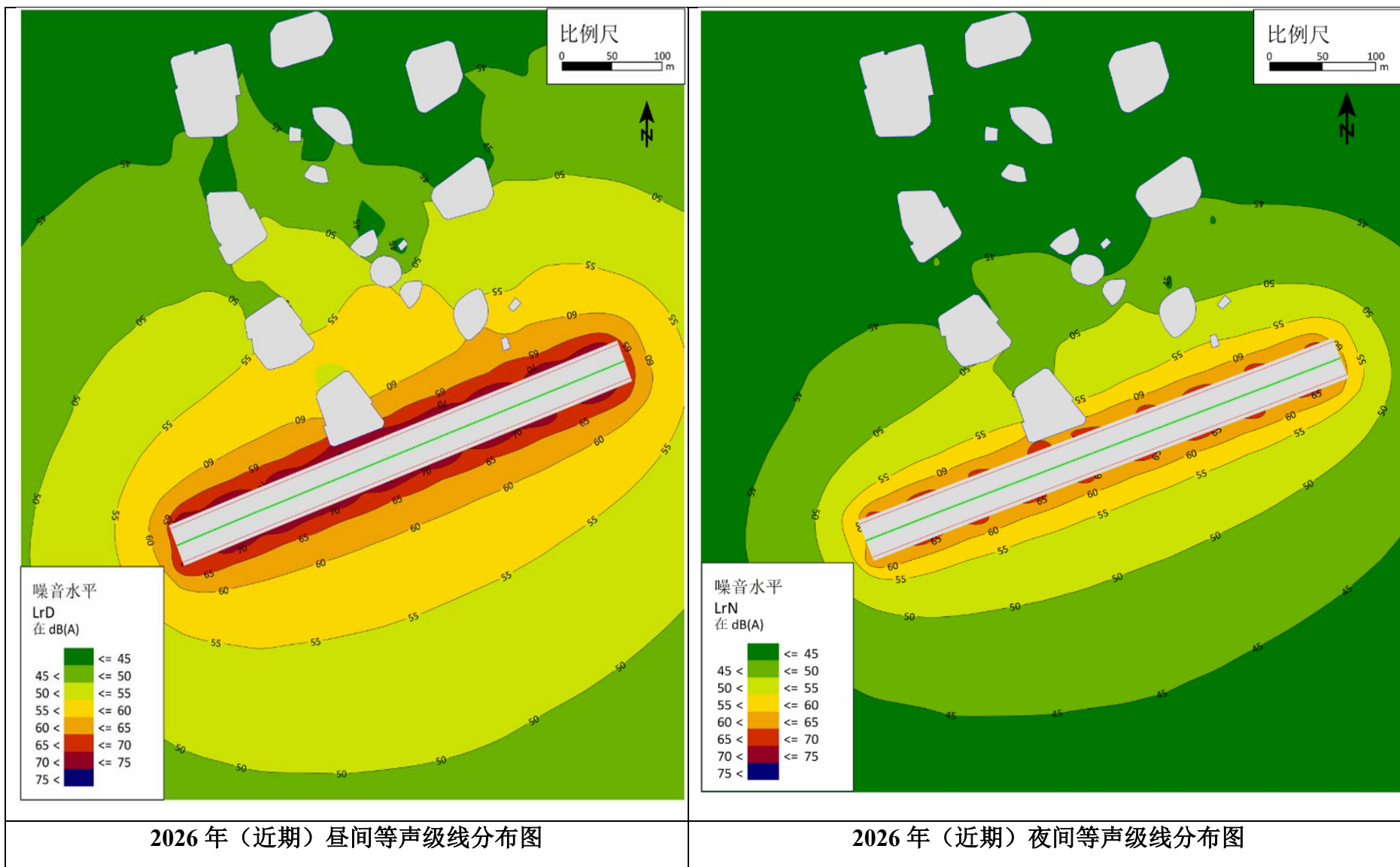
附图 19 项目预测噪声等声线图
