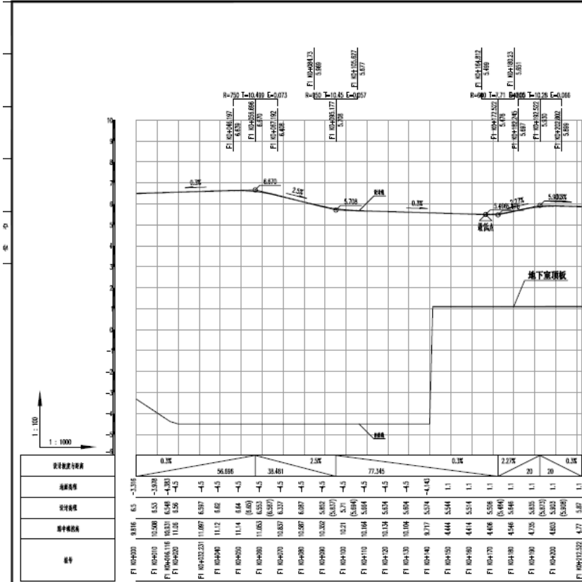
慢行系统纵断面设计图(北侧)
