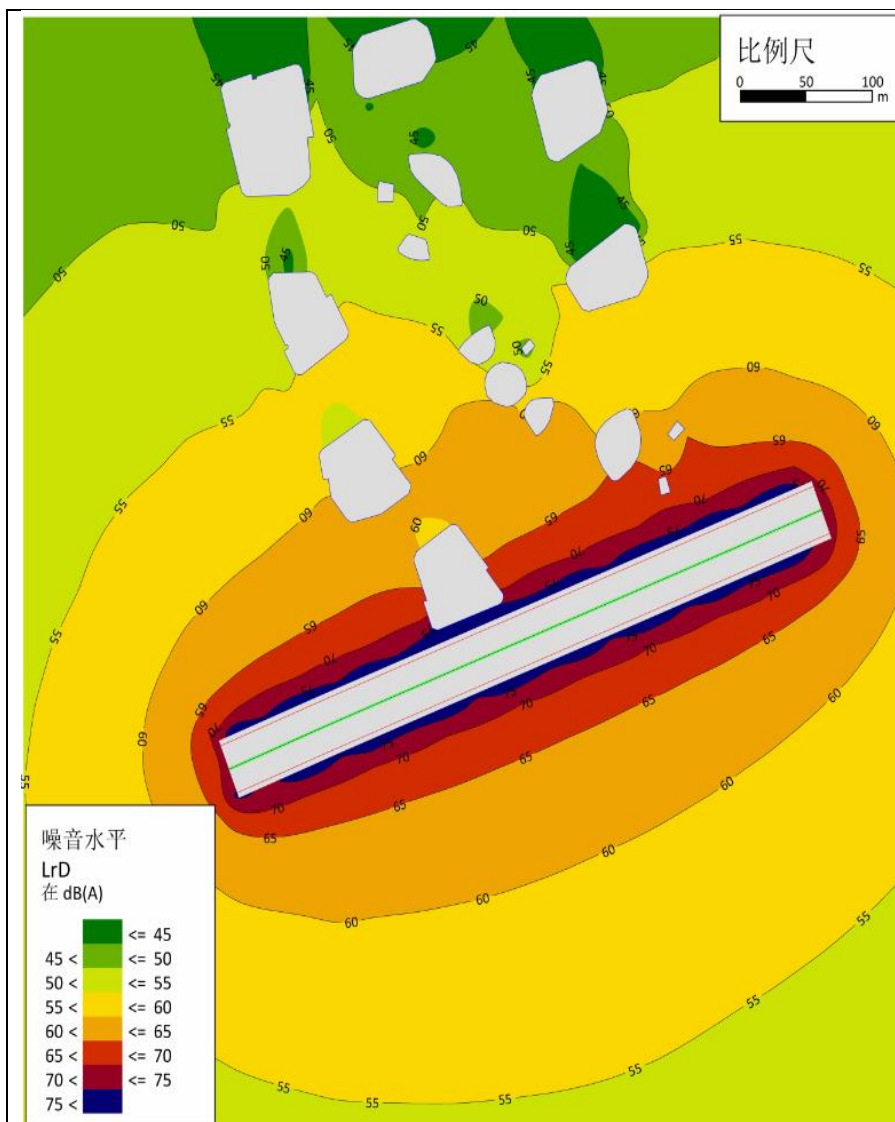
2035 年（中远期）昼间等声级线分布图
