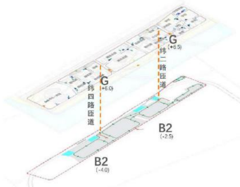
图 2-7 隧道立体图
