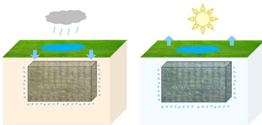
图 2-11 多孔纤维棉模块调蓄雨水蓄水、旱时补水示意图
