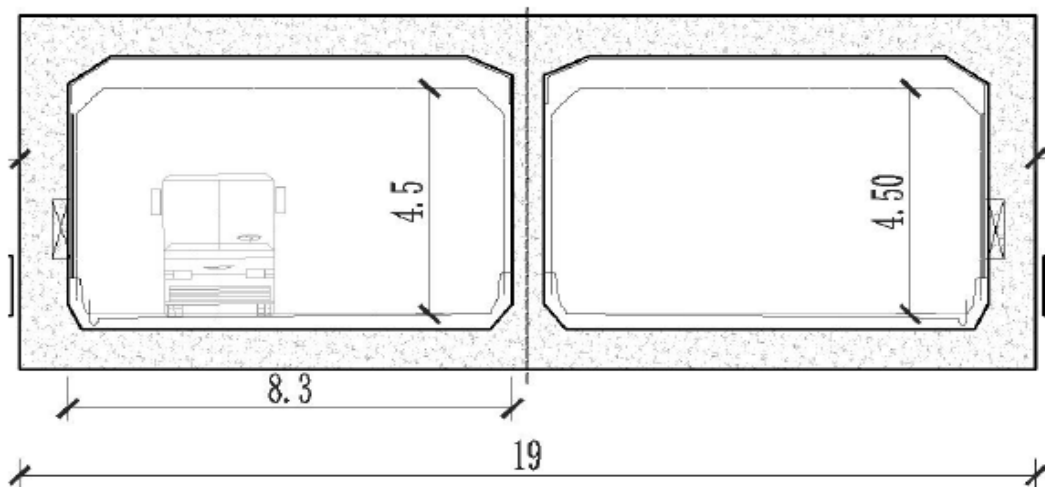
图 2-10 闭口段断面图
