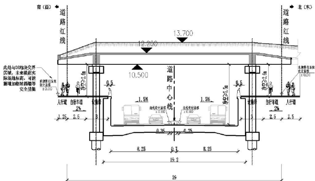
图 2-9 敞口段断面图
