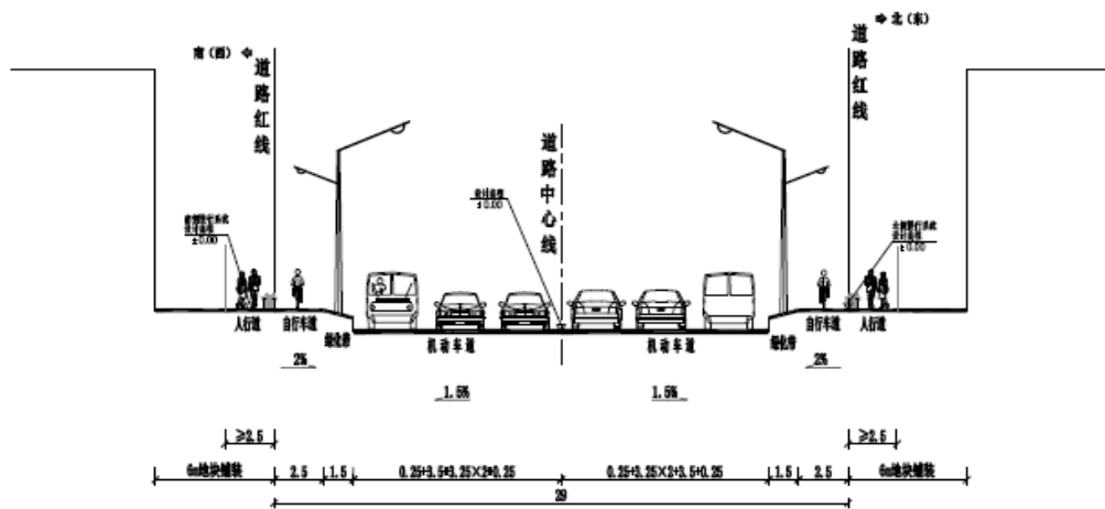
图 2-5 横断面图
