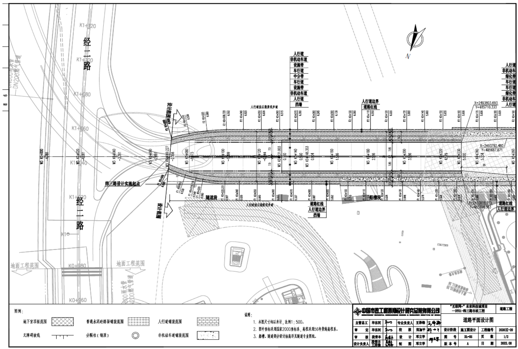
附图16 纬三路道路平面设计图
