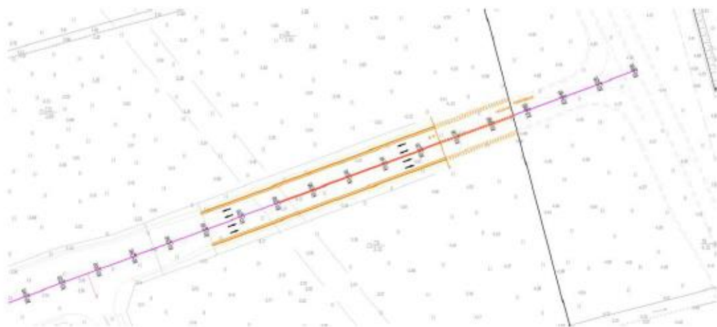
图 2-8 隧道平面图
