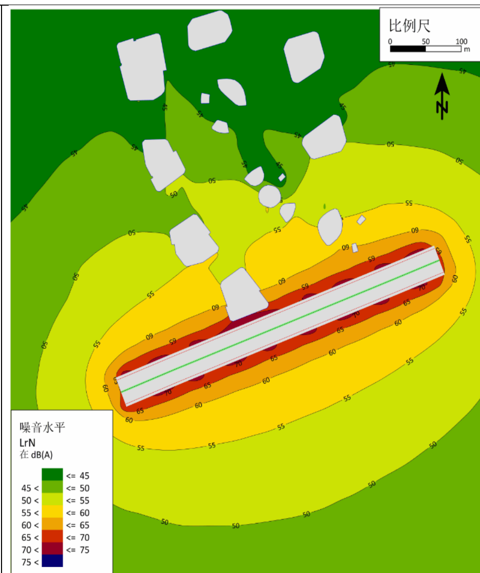
2035 年（中远期）夜间等声级线分布图
